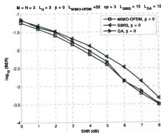
شکل ۱۲- مقایسه‌ی روش های MIMO-OFDM و SBR2 با روش پیشنهادی از نظر نرخ خطای بیت وقتی L_H = 3 و M = N = 3
