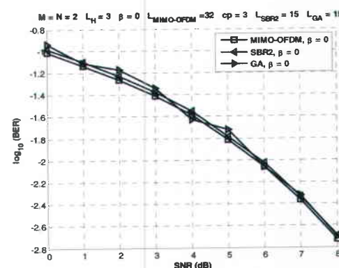
شکل ۱۱- مقایسه‌ی روش های MIMO-OFDM و SBR2 با روش پیشنهادی از نظر نرخ خطای بیت وقتی L_H = 3 و M = N = 2
