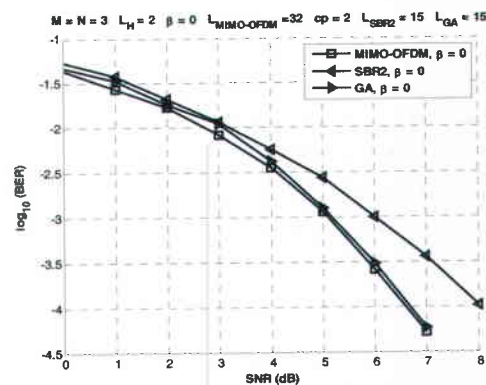
شکل ۱۰- مقایسه‌ی روش های MIMO-OFDM و SBR2 با روش پیشنهادی از نظر نرخ خطای بیت وقتی L_H = 2 و M = N = 3
