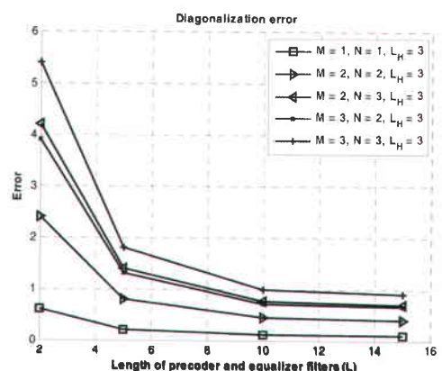
شکل ۷- منحنی خطای همسانسازی بر حسب طول فیلترهای همسانساز و پیش‌کدگذار برای طول کانال L_H = 3
