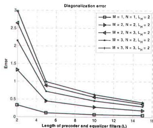
شکل ۶- منحنی خطای همسانسازی بر حسب طول فیلترهای همسانساز و پیش کدگذار برای طول کانال L_H = 2
