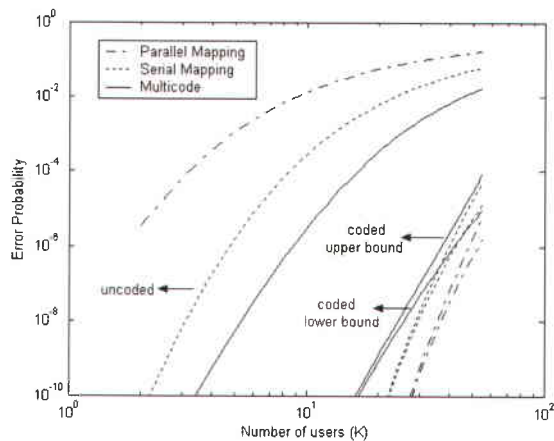
شکل ۵. احتمال خطا بر حسب تعداد کاربران به ازای SNR = 18dB, N_s = 256, N_b = 64
